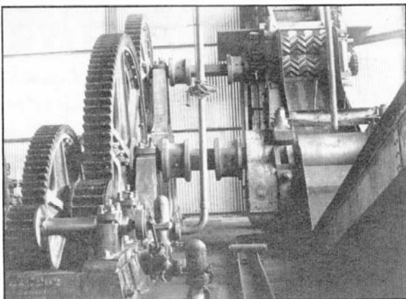
På G.A.Hagemann's plantage LaGrange blev øernes første moderne „cane-crusher“ opstillet. Bemærk de knusende og bidske „tænder“ oppe i højre hjørne
